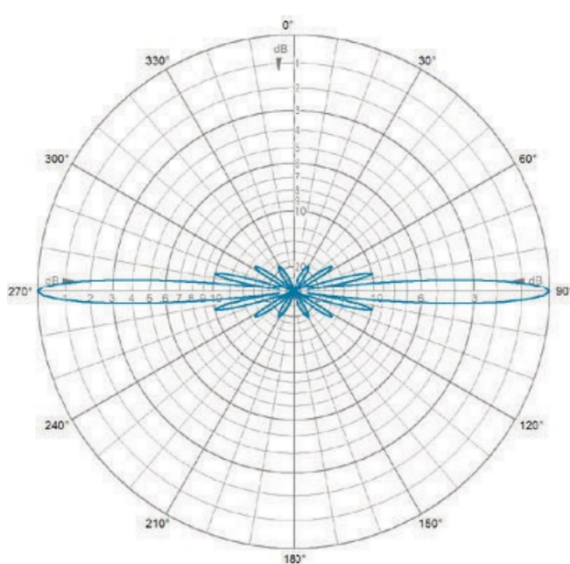
E-Plane | 780 MHz
