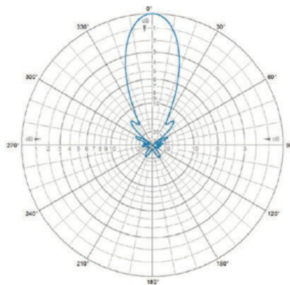
H-Plane | 915 MHz
