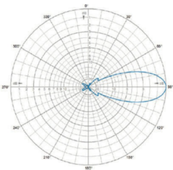
E-Plane | 915 MHz
