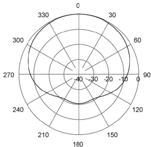
H-Plane | 165 MHz
