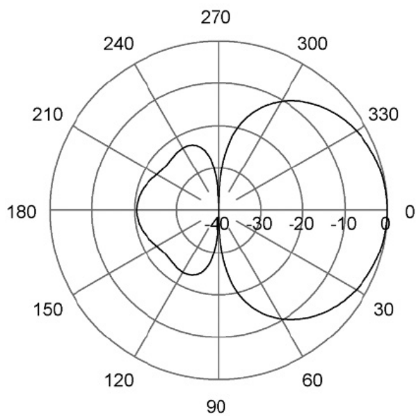
E-Plane | 165 MHz
