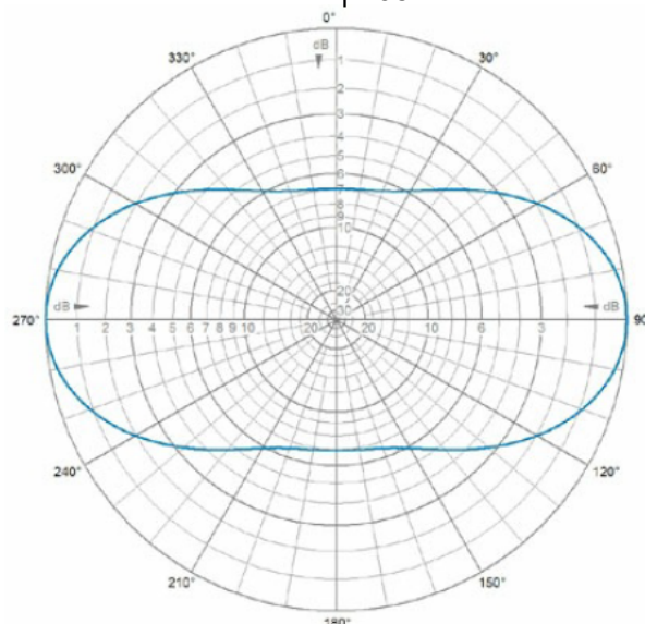
H-Plane | 165 MHZ
