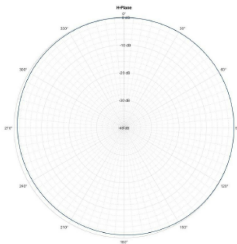
H-Plane, 915MHz
