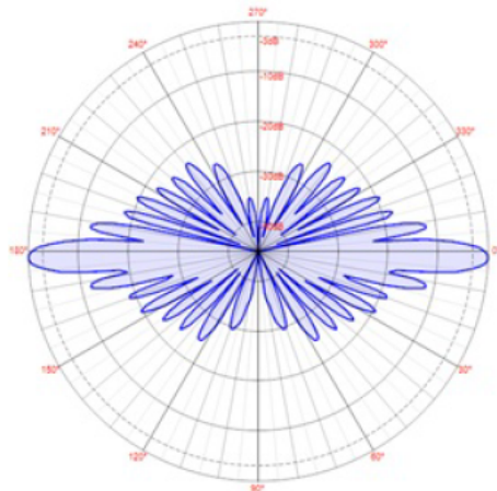
Elevation Pattern, 2°
